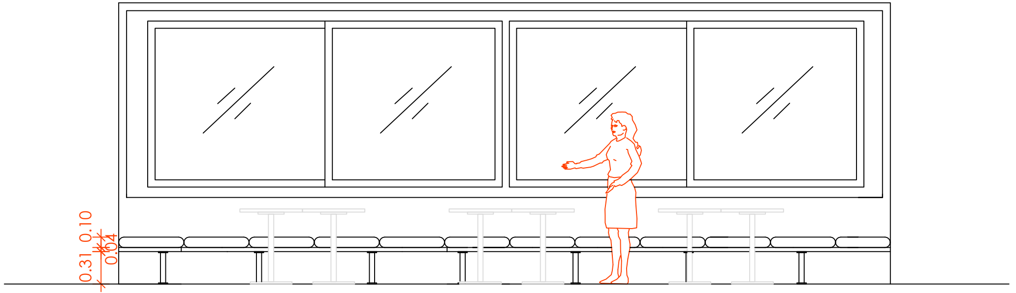
Alçat detall moble 4G
