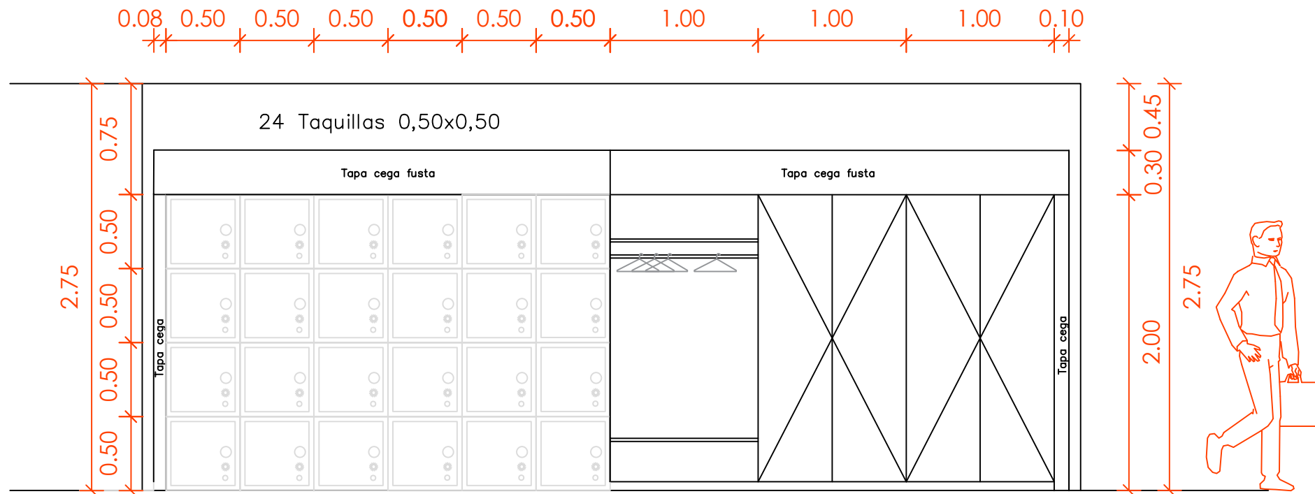
Alçat detall moble 5D
