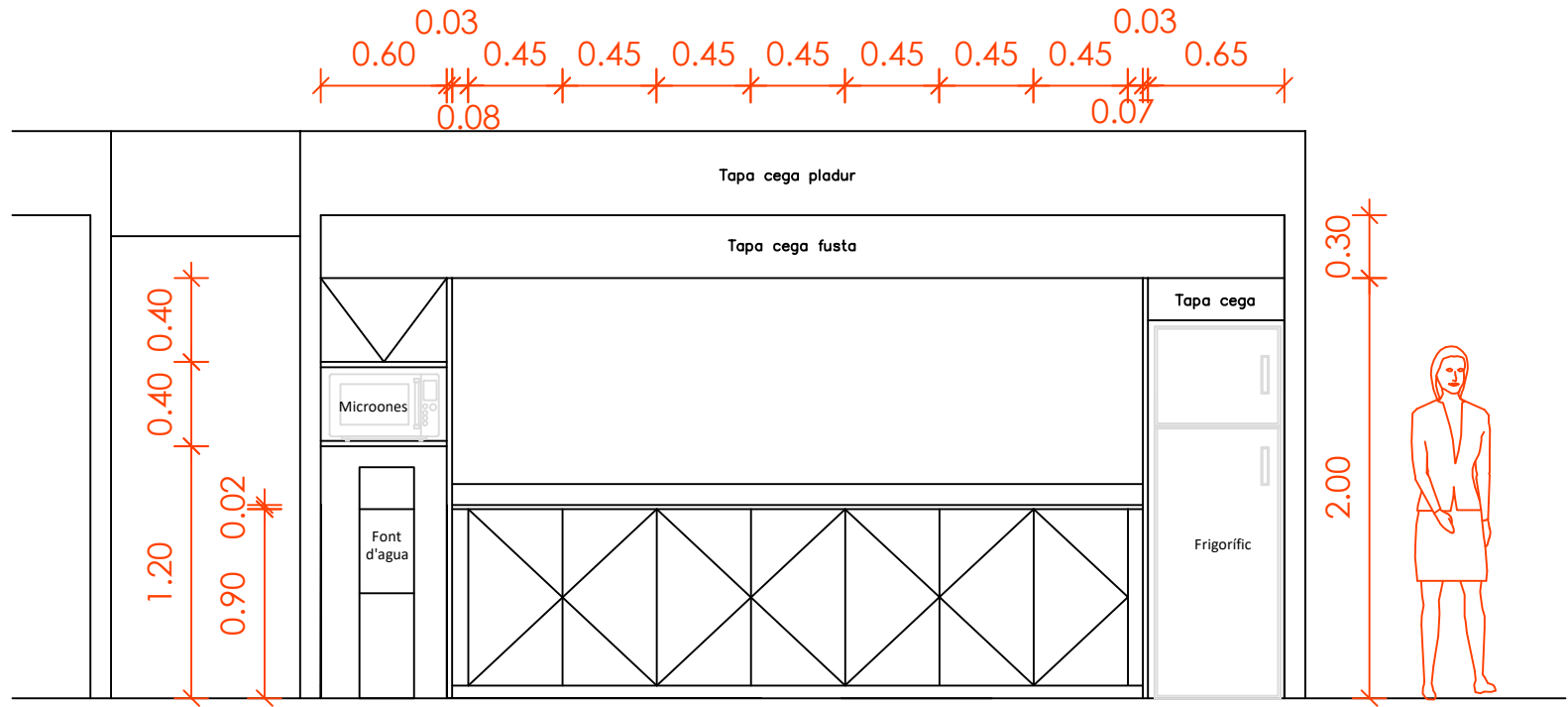
Alçat detall moble 5A
