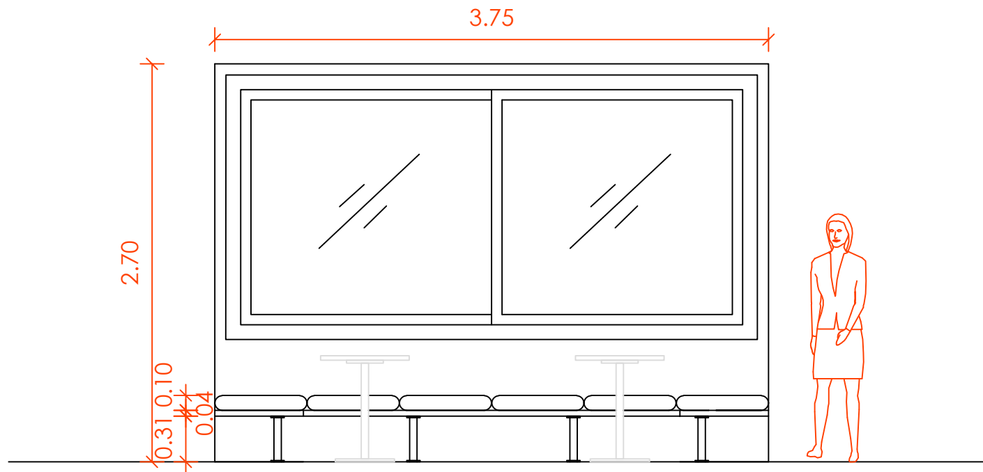
Alçat detall moble 4B
