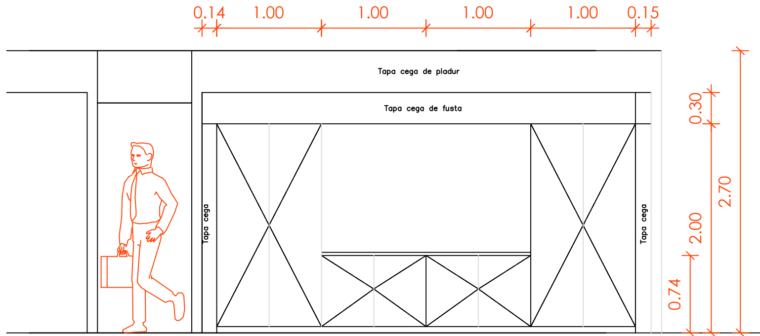
Alçat detali mobil 4A
