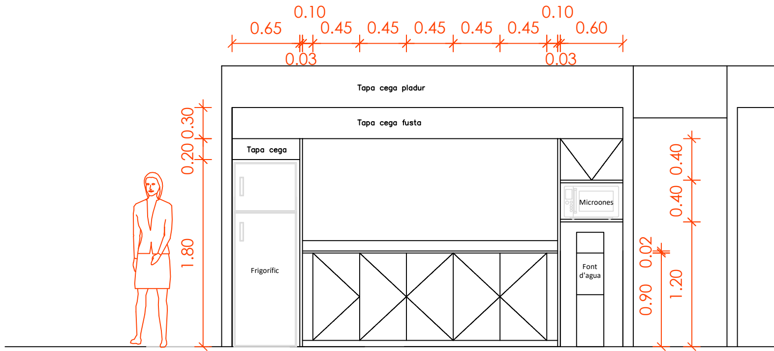
Alçat detall moble 4F
