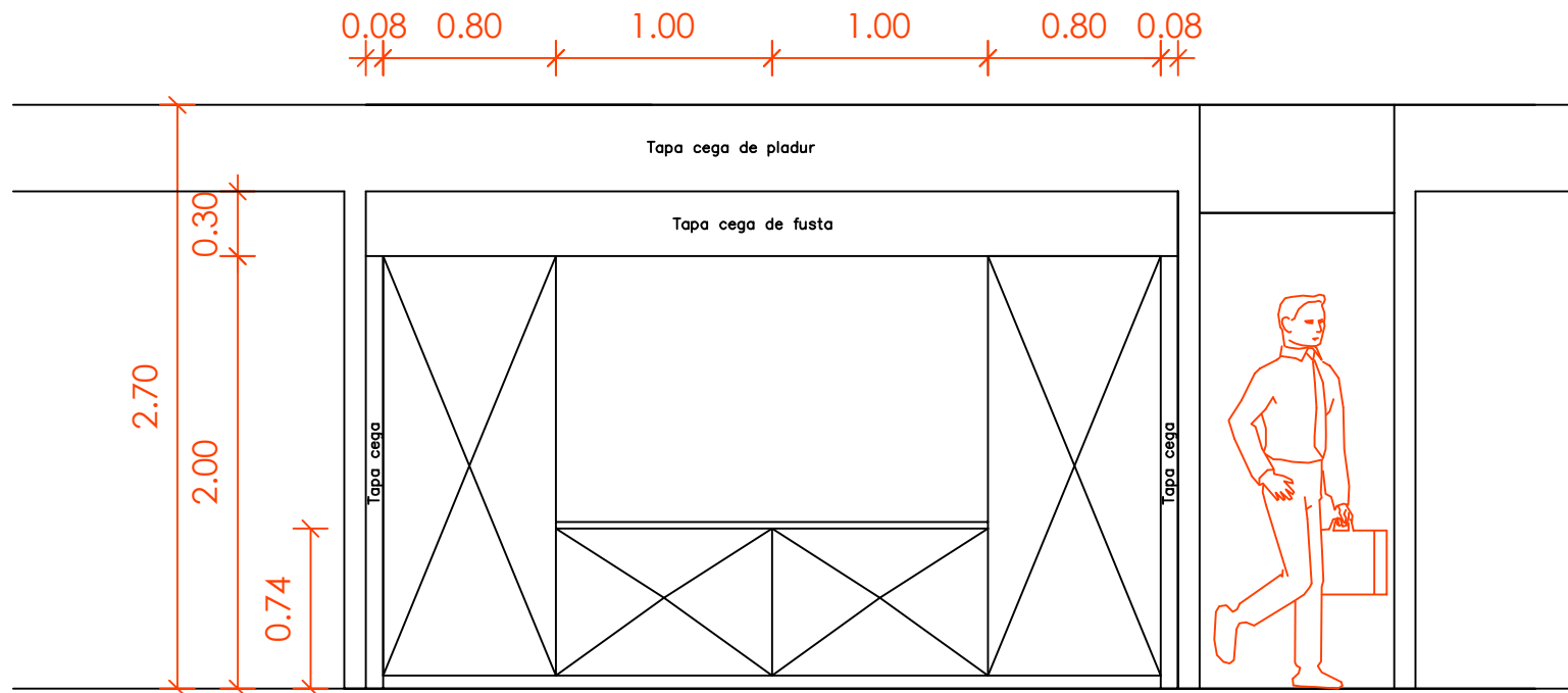
Alçat detall moble 5E
