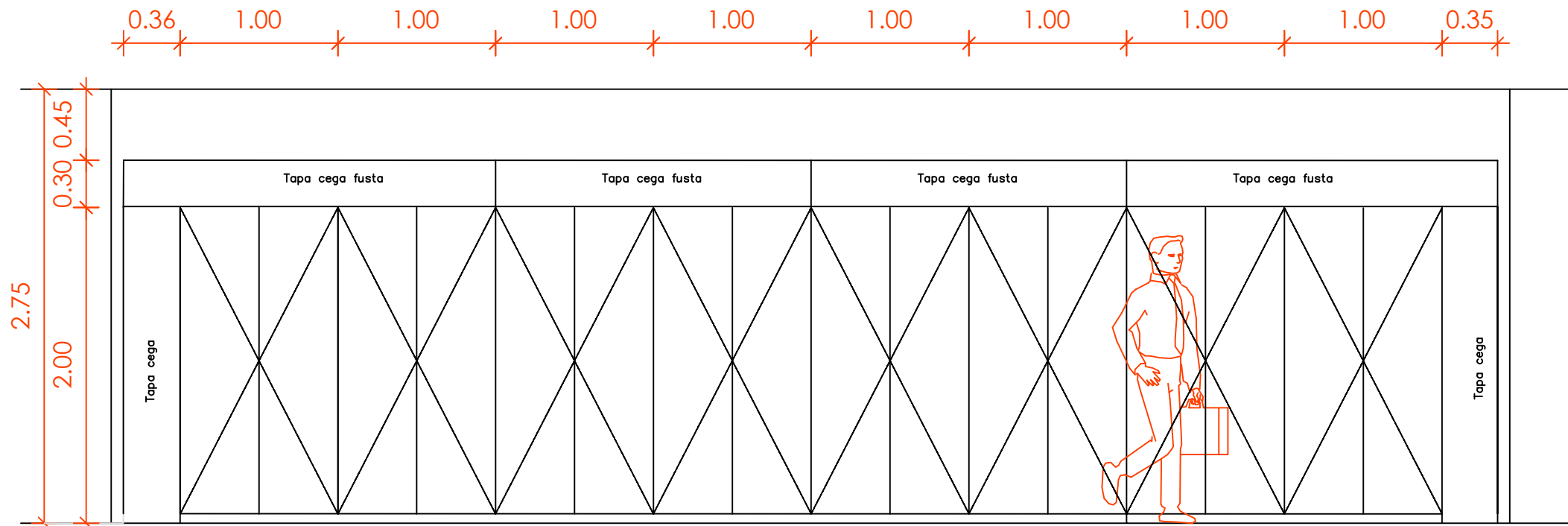
Alçat detall moble 4D
