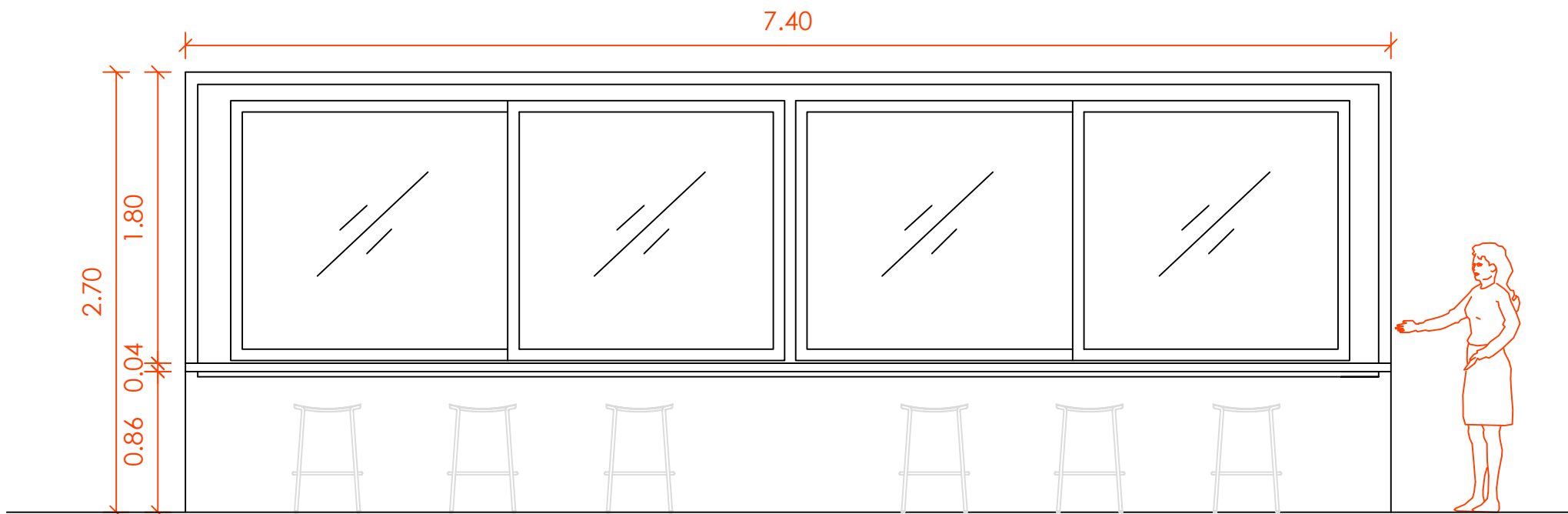
Alçat detall moble 5F
