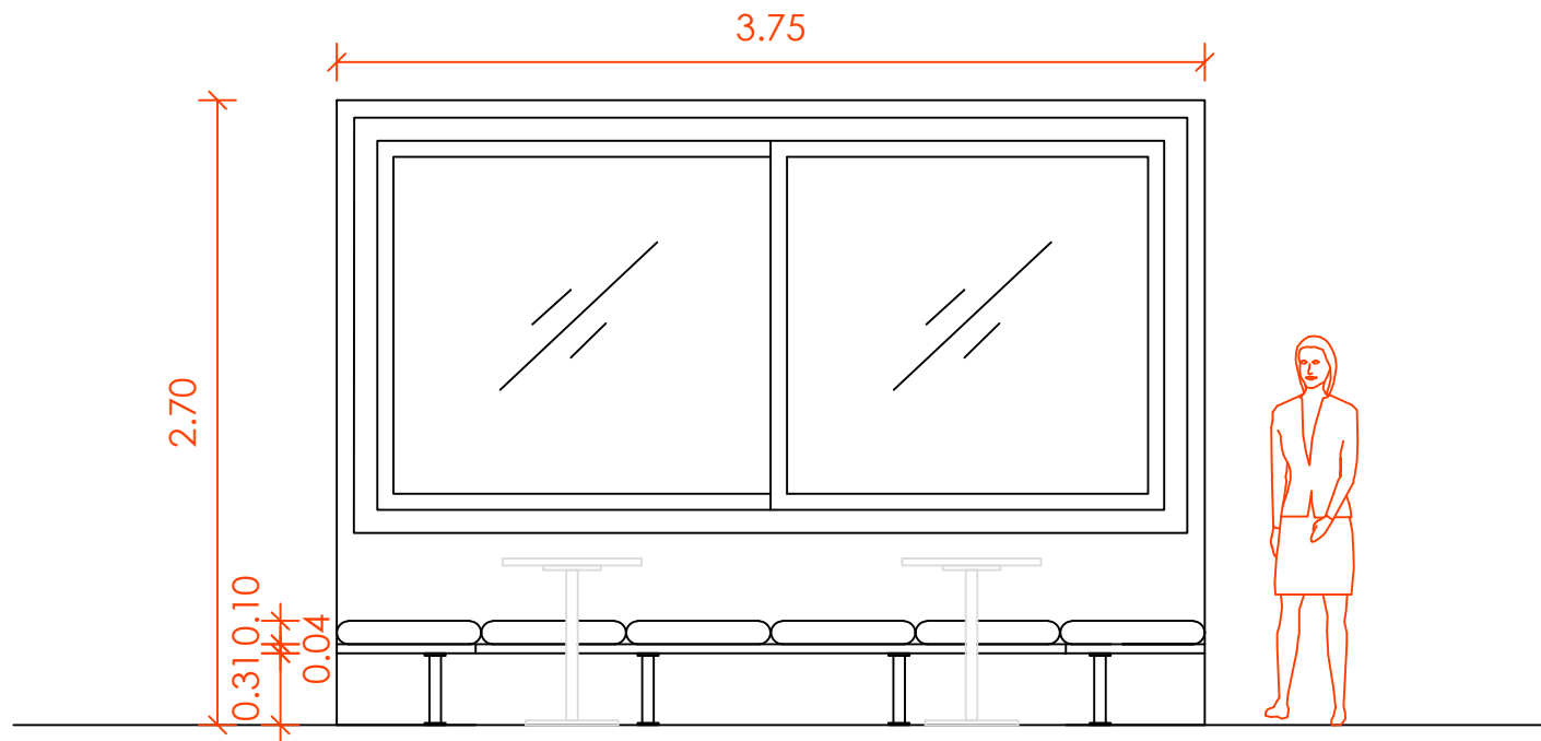
Alçat detall moble 5B
