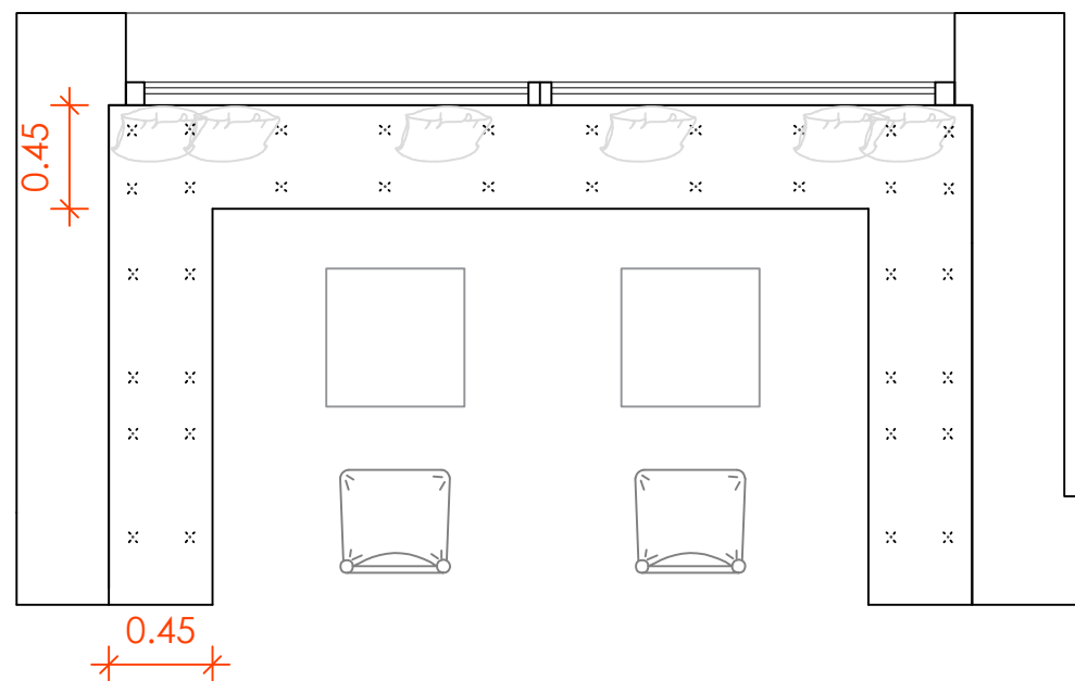
Planta detall moble 4B
