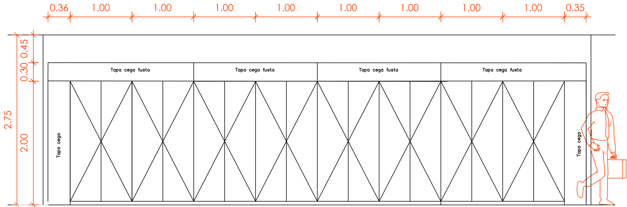
Alçat detall moble 5C
