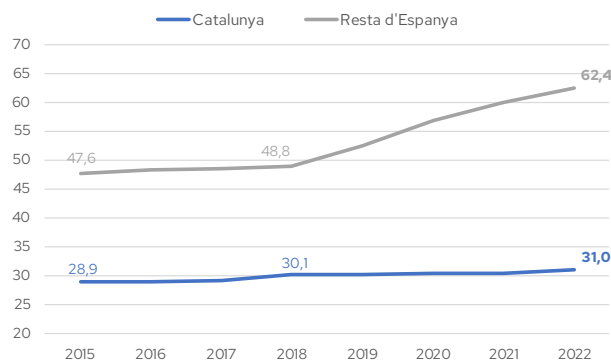
Gràfic 5.A. Estoc de potència d'energia elèctrica renovable. % sobre potència elèctrica instal·lada total
